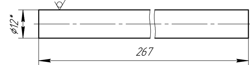
Дет. поз. 1.1 (1:1)
