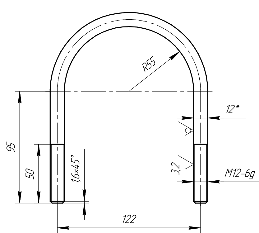
Дет. поз. 3 (1:2)
