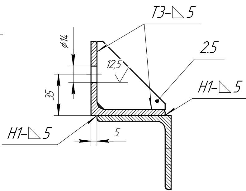
В-В(1:2)
