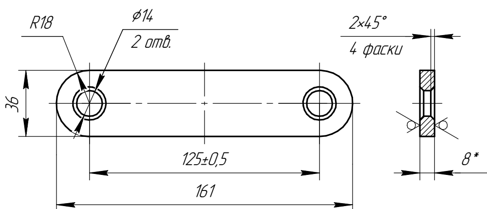
Дет. поз. 1.4 (1:2)
