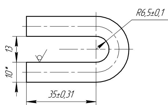
Дет. поз. 1.3 (1:1)
