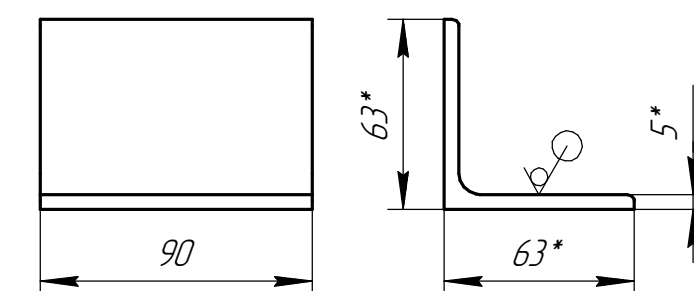
Дет. поз. 2.2 (1:2,5)
