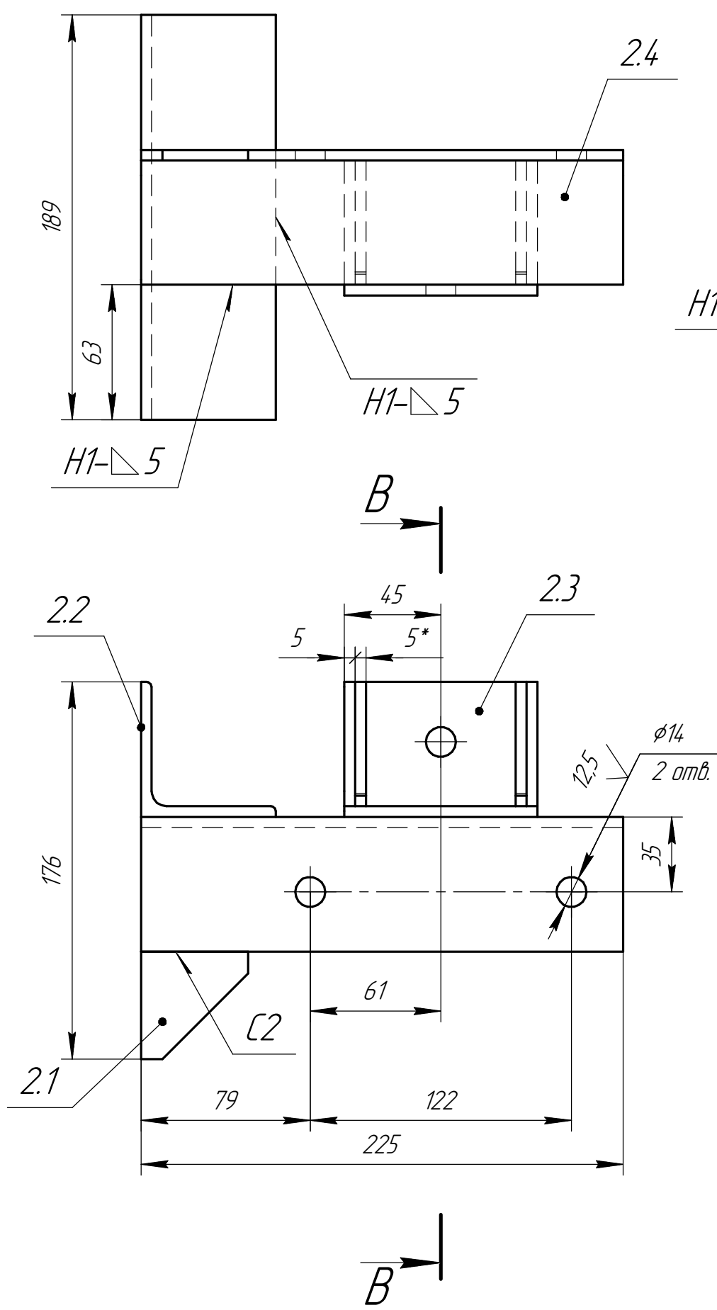
Дет. поз. 2 (1:2,5)
