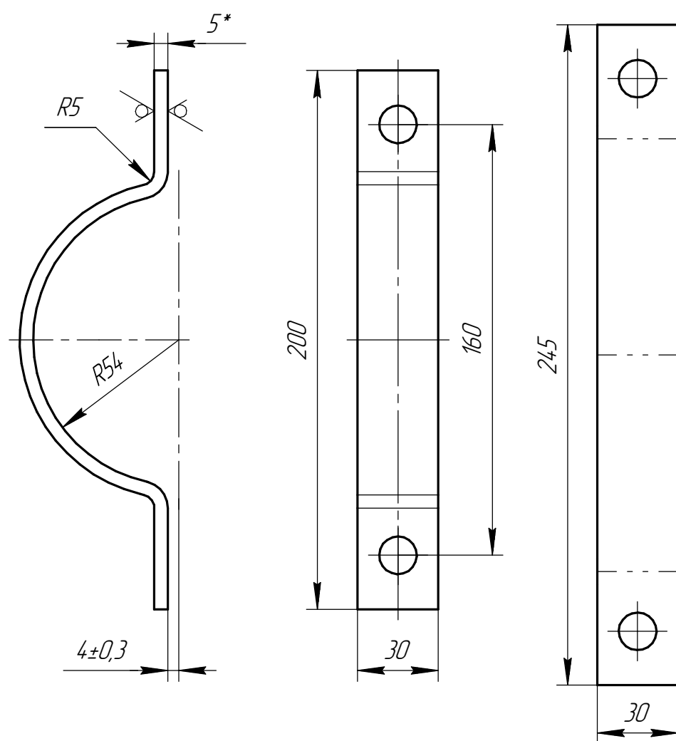
Дет. поз. 1.5 (1:2)
