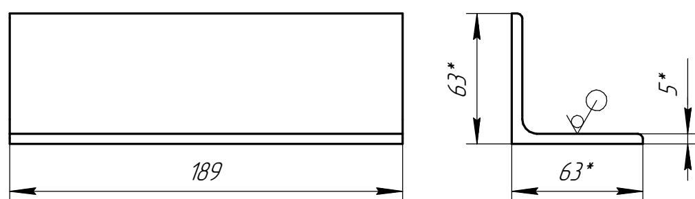
Дет. поз. 2.4 (1:2,5)
