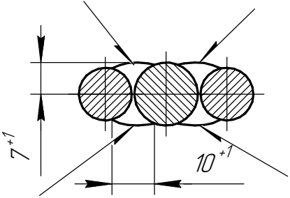
Б-Б(1:1)
