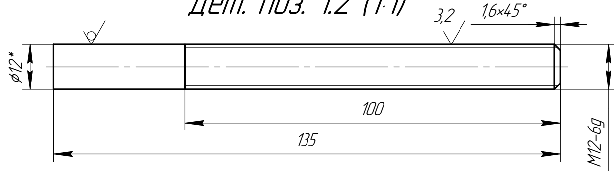
Дет. поз. 1.2 (1:1)
